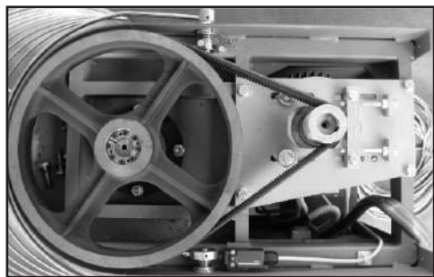
Стандартная трансмиссия
