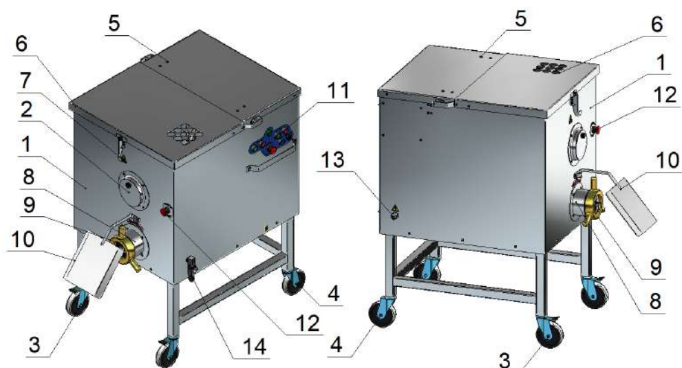
Рис. 1 Устройство мясорубки
