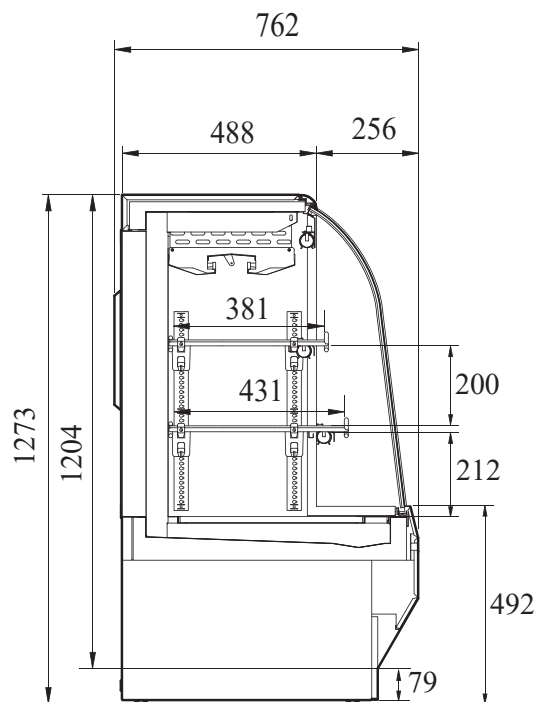
ВИД СБОКУ
