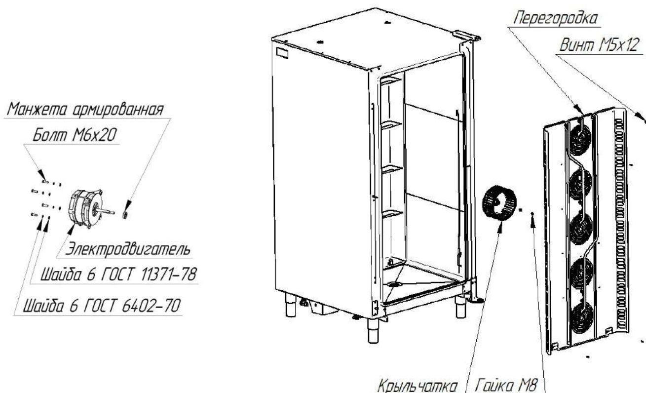
Рис. 11. Замена манжет
