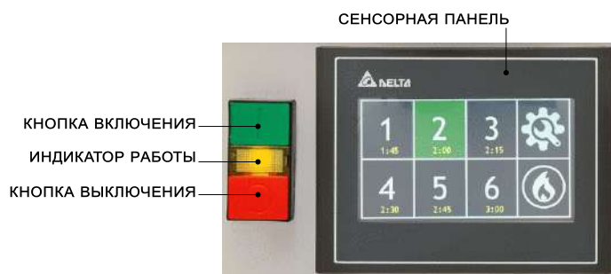
Рисунок 2: Панель управления
