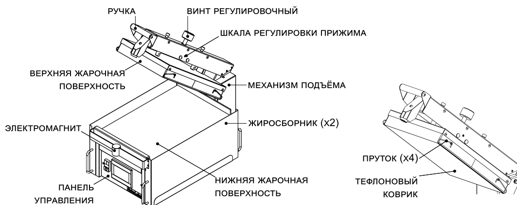
Рисунок 1: Основные компоненты
