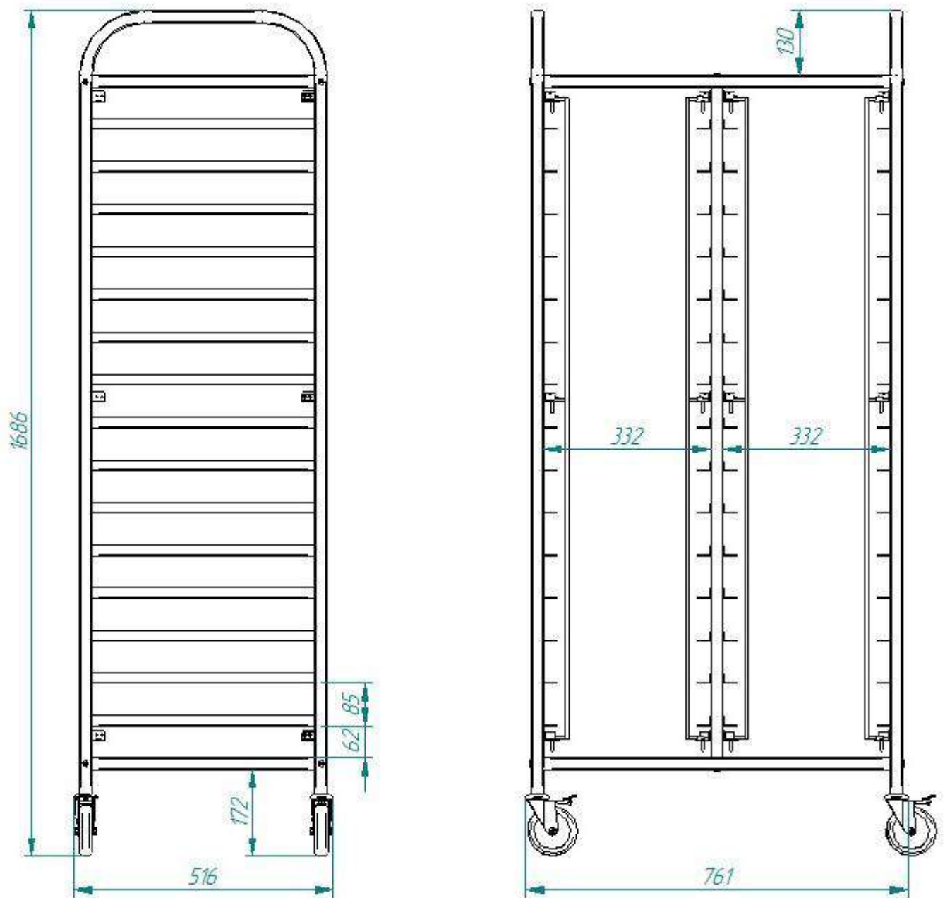
Рис.1 Общий вид
