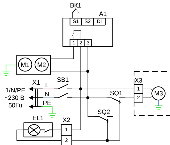
Схема электрическая принципиальная ШХс-1,4-02, ШХс-1,4-03
