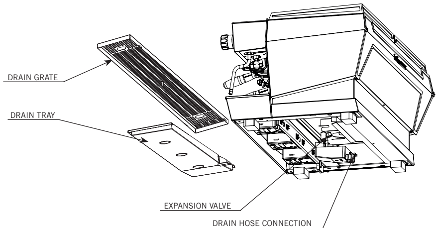
Fig. 3 - Installation Nomenclature
