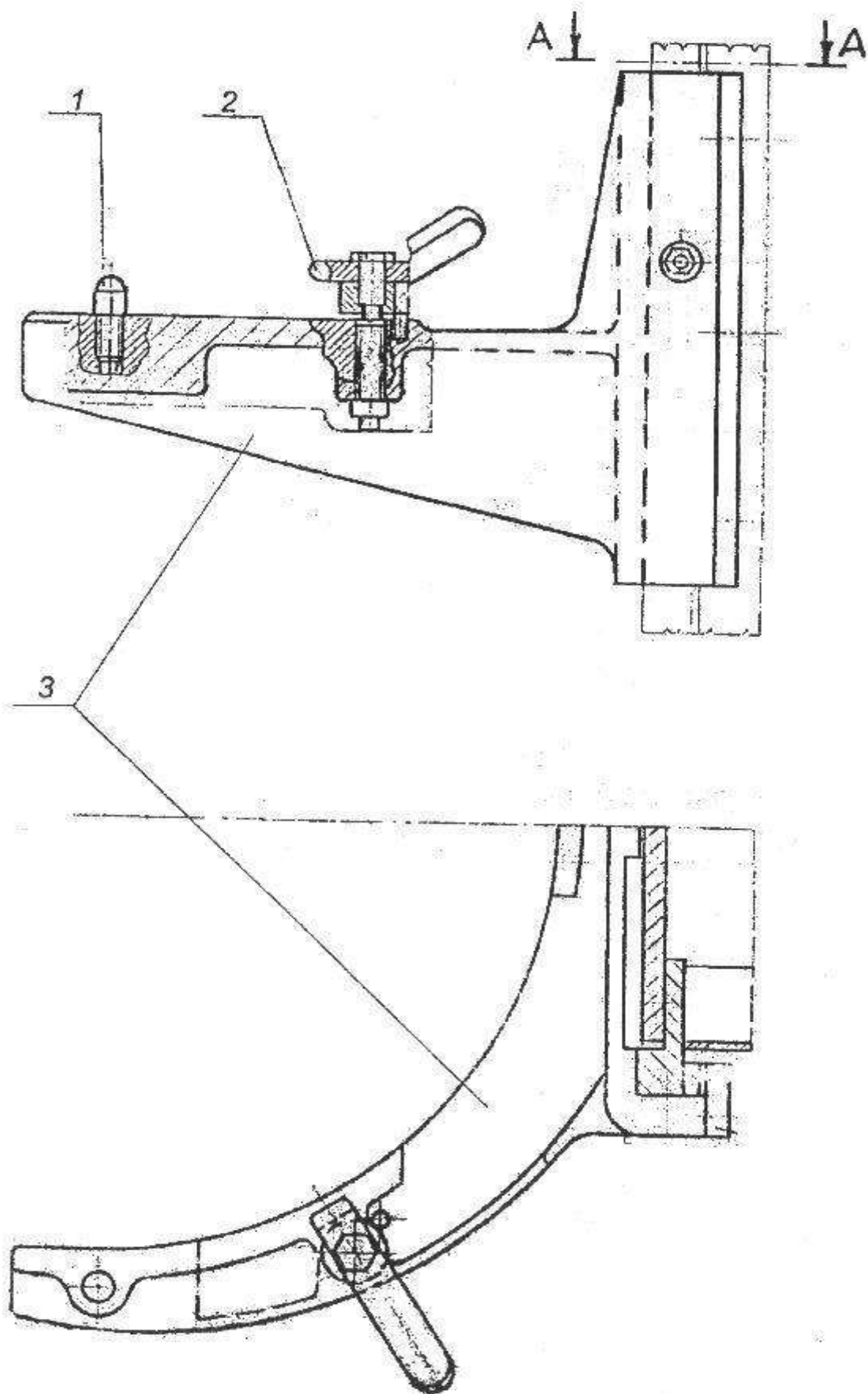
Рисунок 4 А-А 1.Фиксатор; 2. Зажим; 3.Корпус стола.
