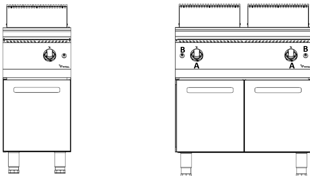
Рис. 1. ПАНЕЛЬ УПРАВЛЕНИЯ
