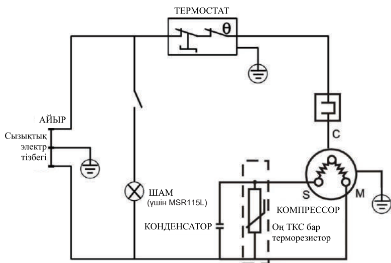
Электр схемасы
