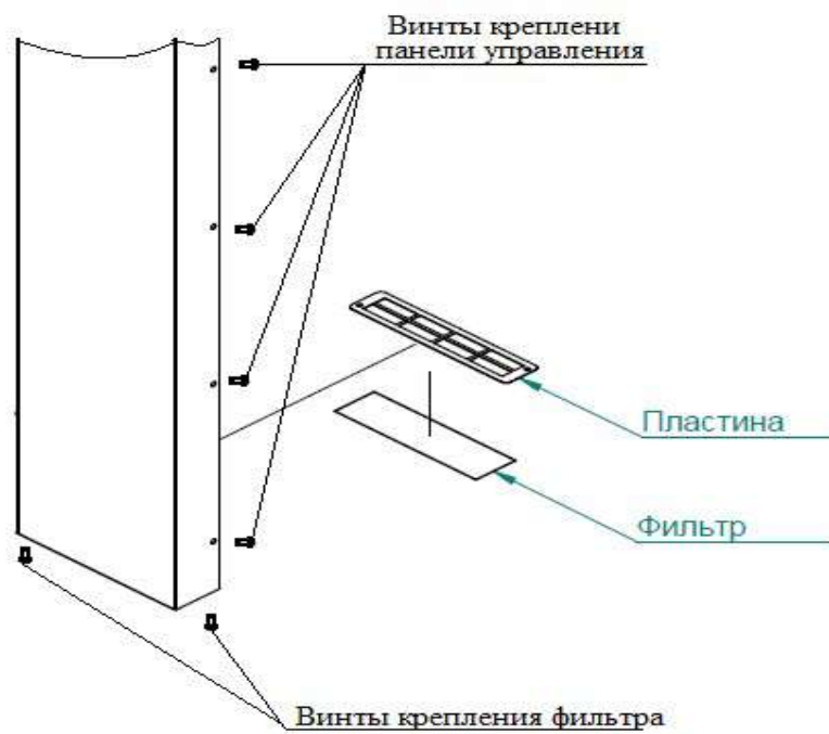
Рис. 17. Замена фильтра
