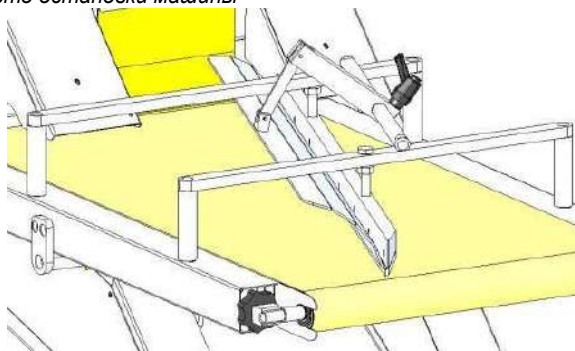
Рисунок 18: Установка угла округлителя
