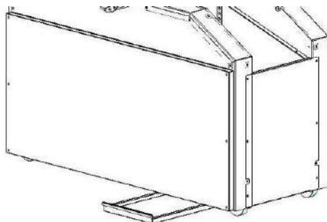
Рисунок 12: Установка машины
