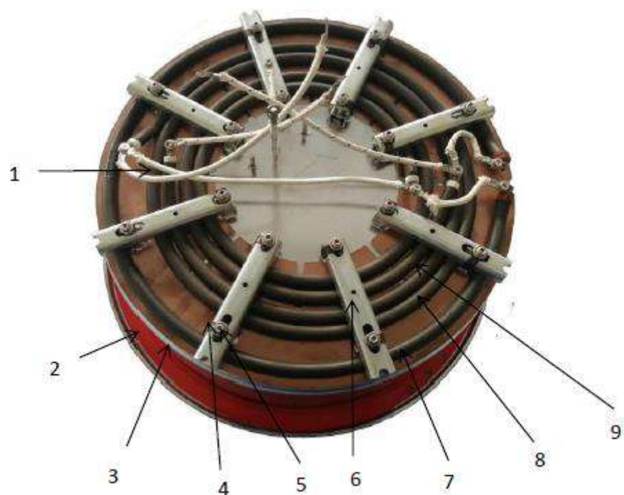
Нагревательный элемент
