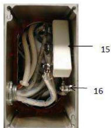
Соединительная коробка
