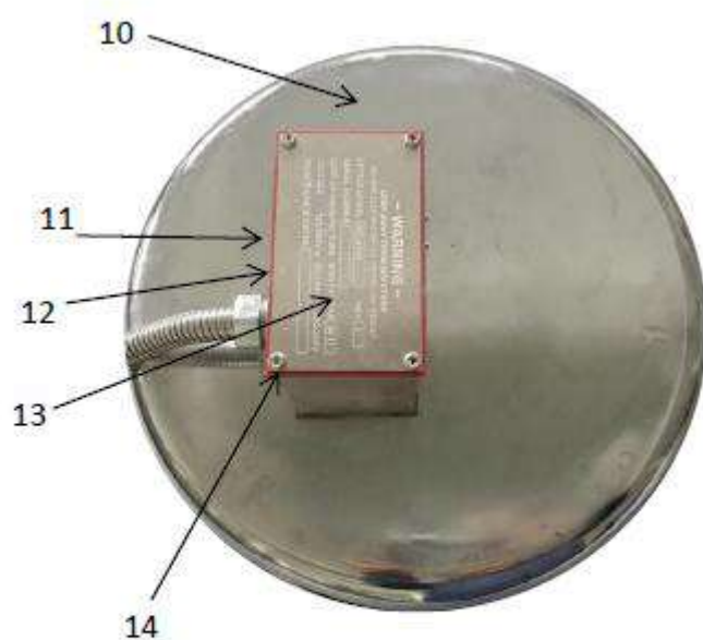
Днище
