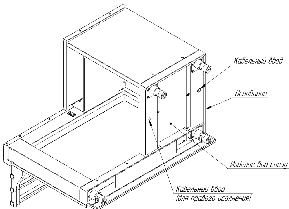
Рис.1 Схема возможного подвода электропитания к изделию КК-70Е.
