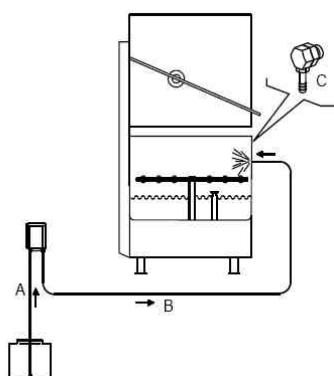
СХЕМА ПОДСОЕДИНЕНИЯ
