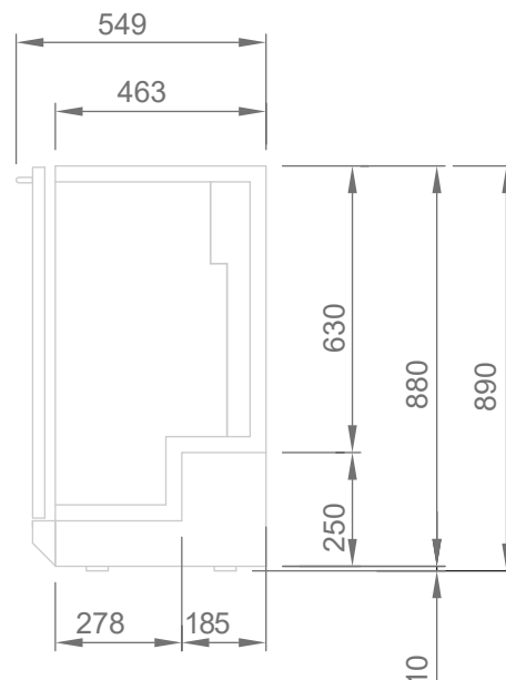
ВИД СБОКУ
