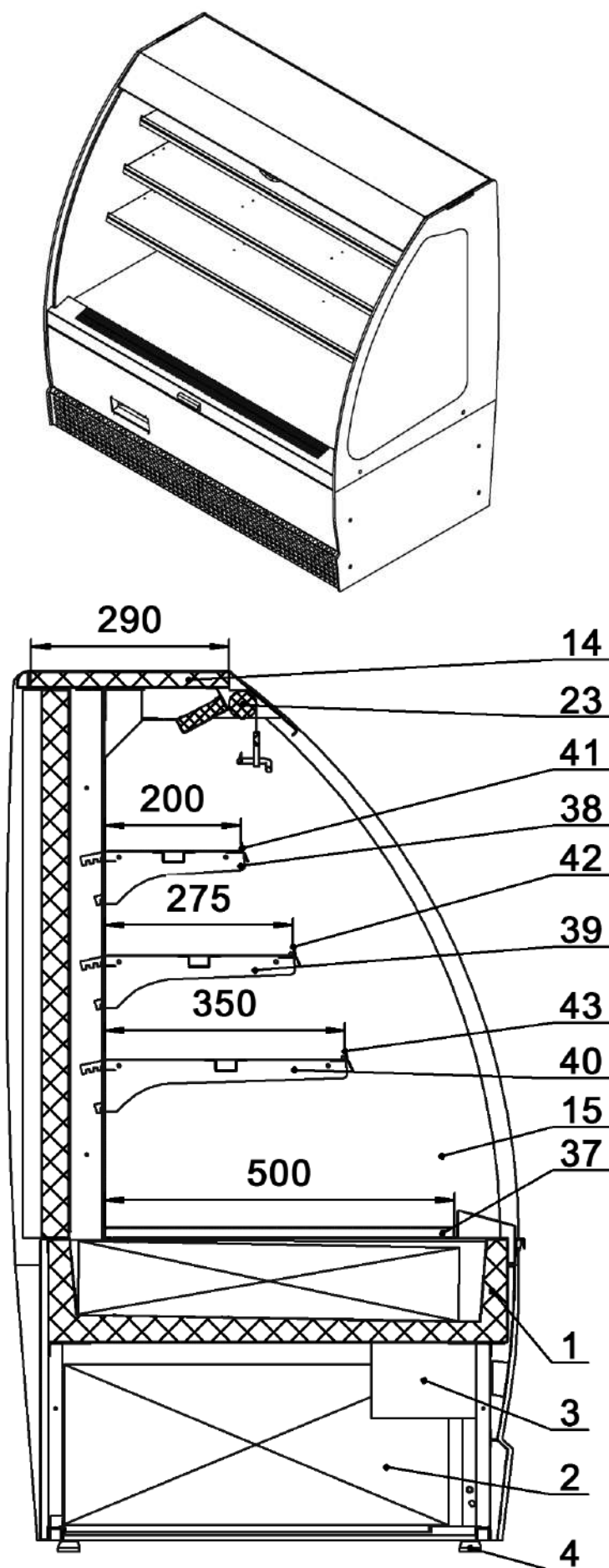
Схема сборки VSo-0,95GK / 1,3GK
