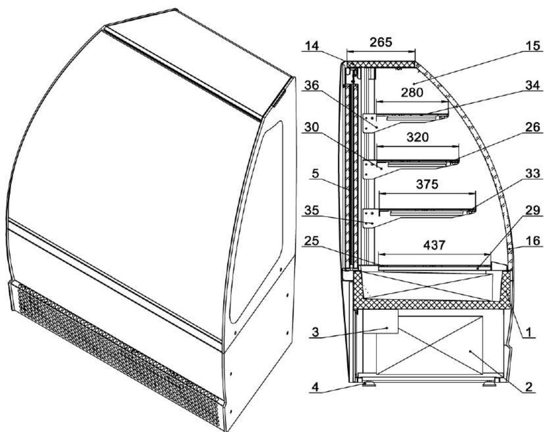
Схема сборки VS-UN
