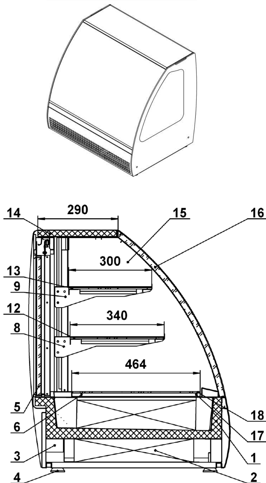
Схема сборки VSn-0,95
