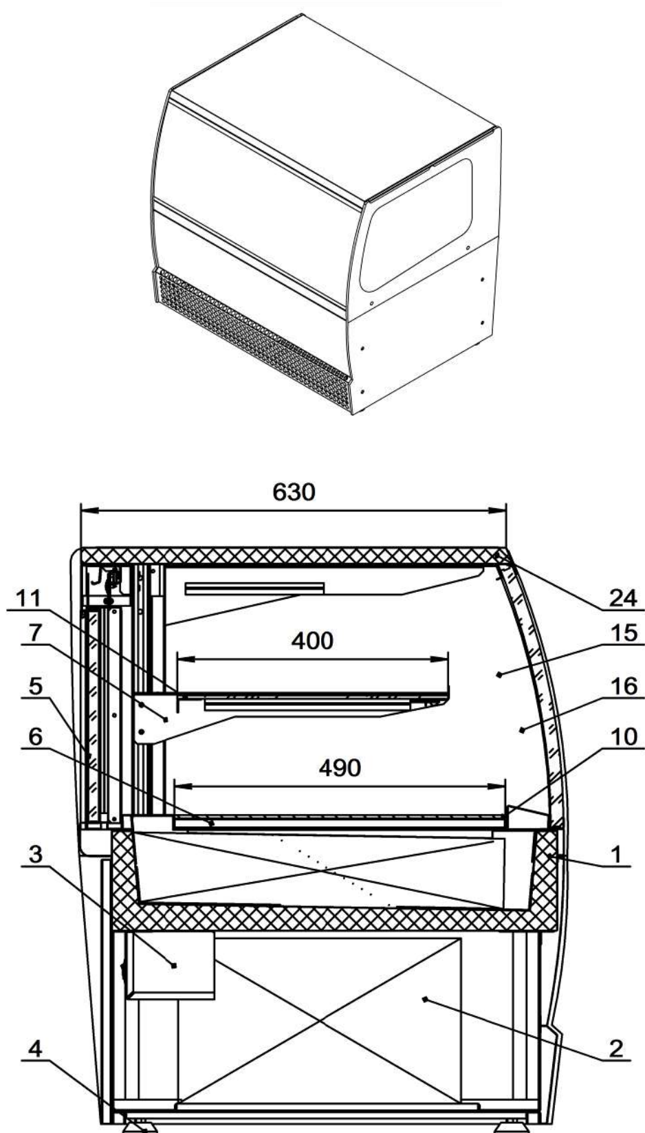
Схема сборки VSk-0,95
