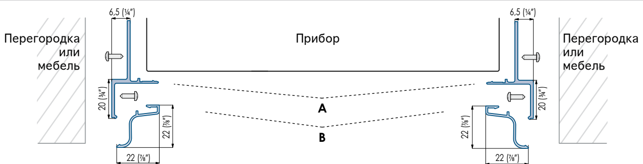
А- Профиль бокового соединения
