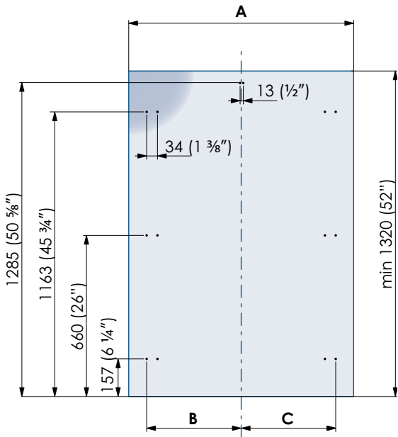
Расположение отверстий
