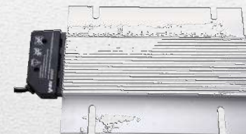
Нагревательный элемент 305 для мармита 721R61-1 0,35 кВт, 220В
